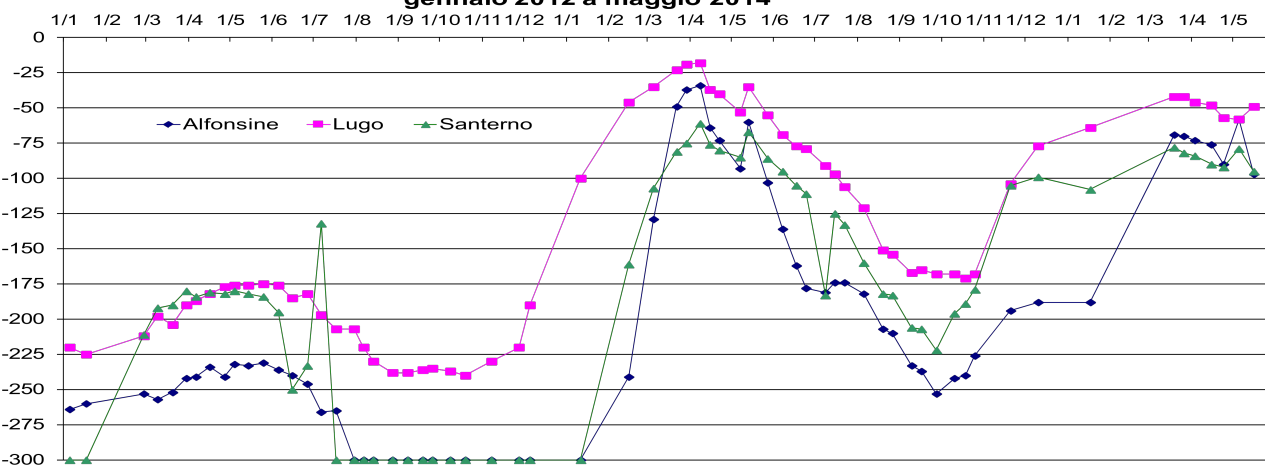
Evoluzione della profondità di falda in 3 località della provincia di Ravenna da gennaio 2012 a maggio 2014
